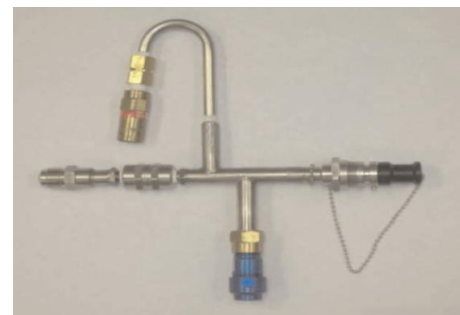
LOX-Füllpistole
